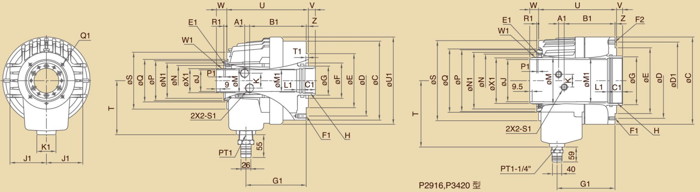
寸法図 >> Dimensions
